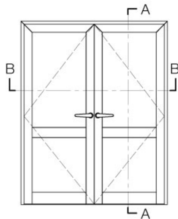
ELEVATION
