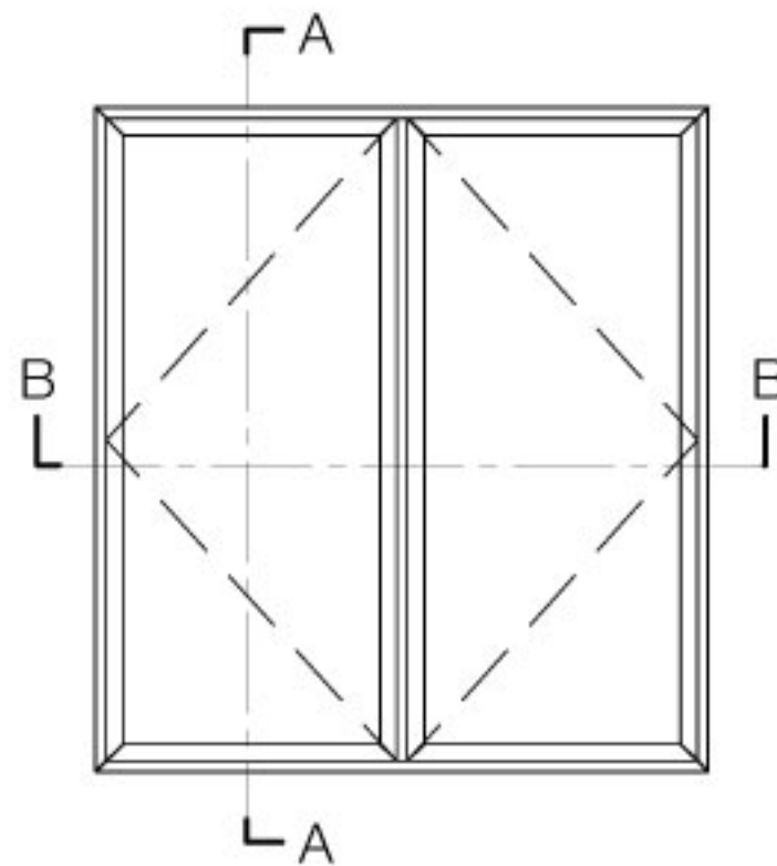
ELEVATION
