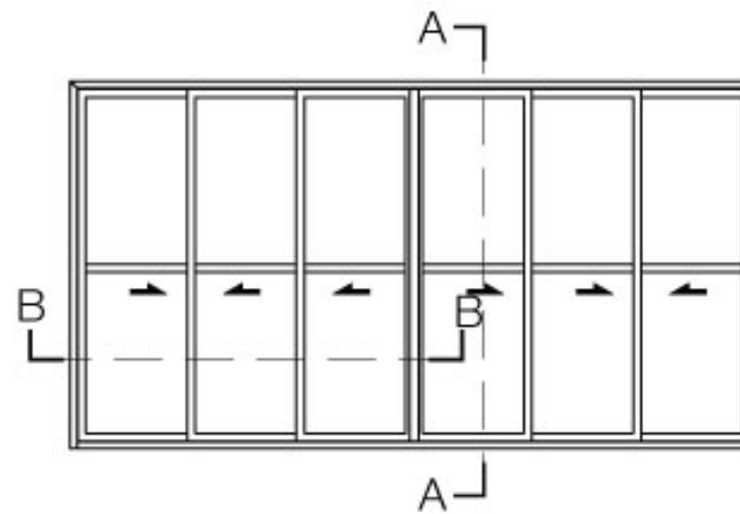
ELEVATION
